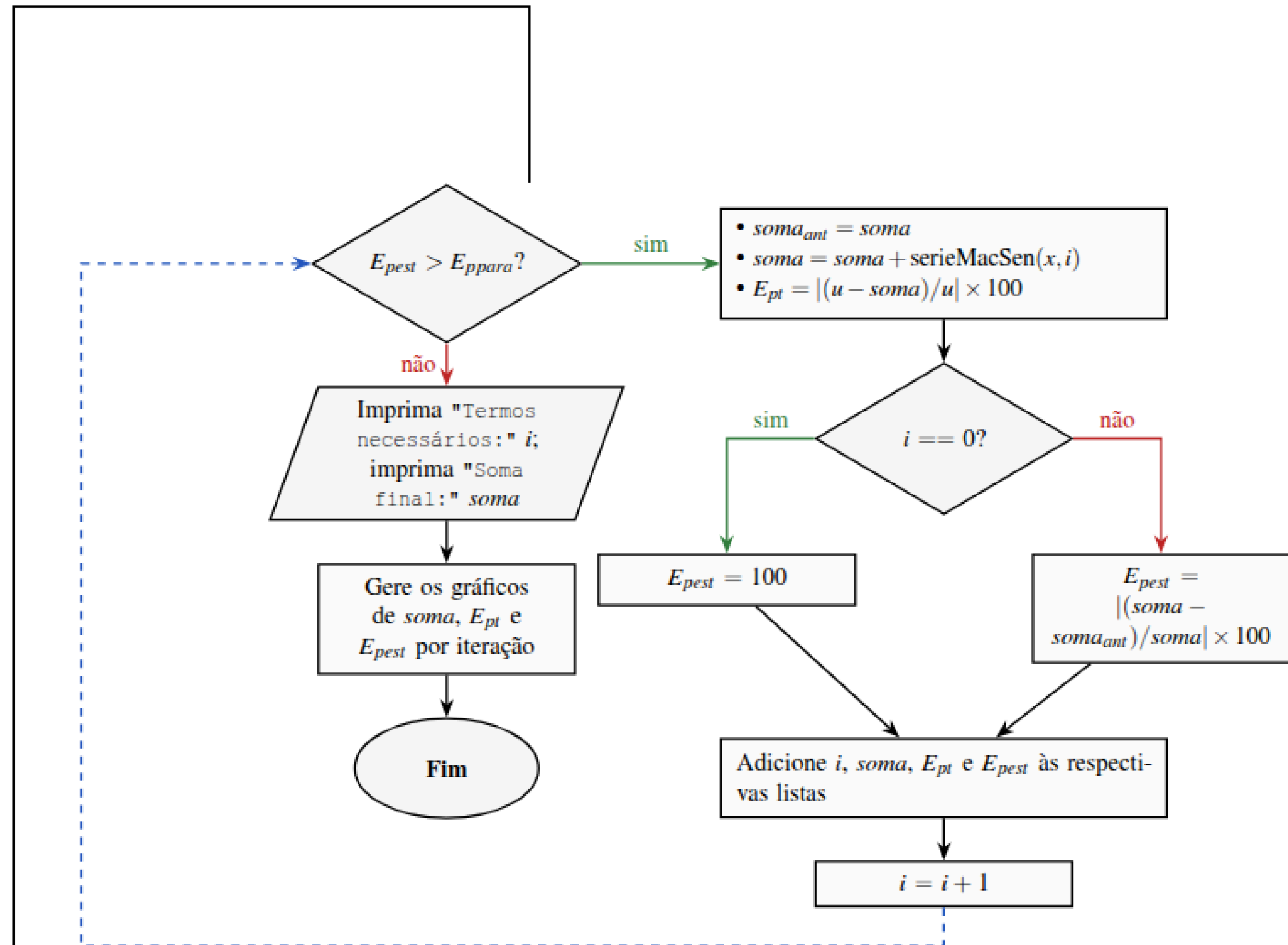
Figura 2: Fluxograma do algoritmo para estimar \text{sen}(x) por série de Maclaurin
